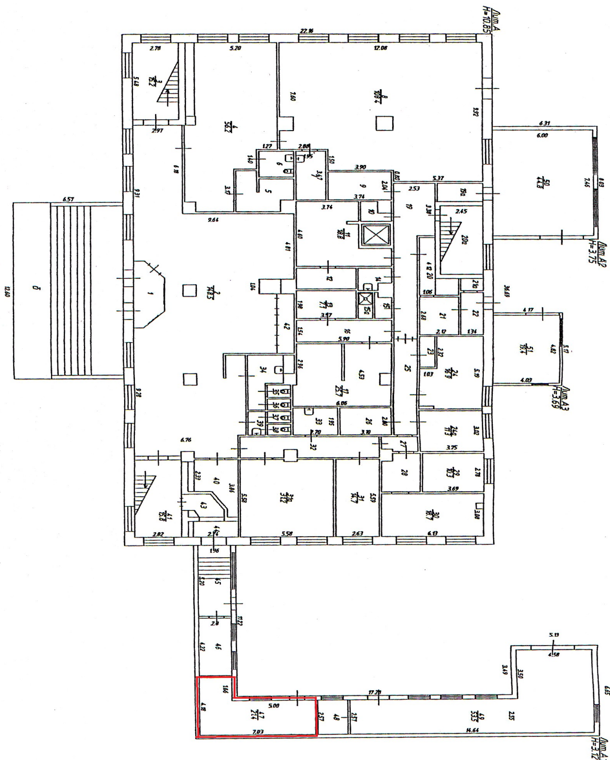
План 1 этажа
