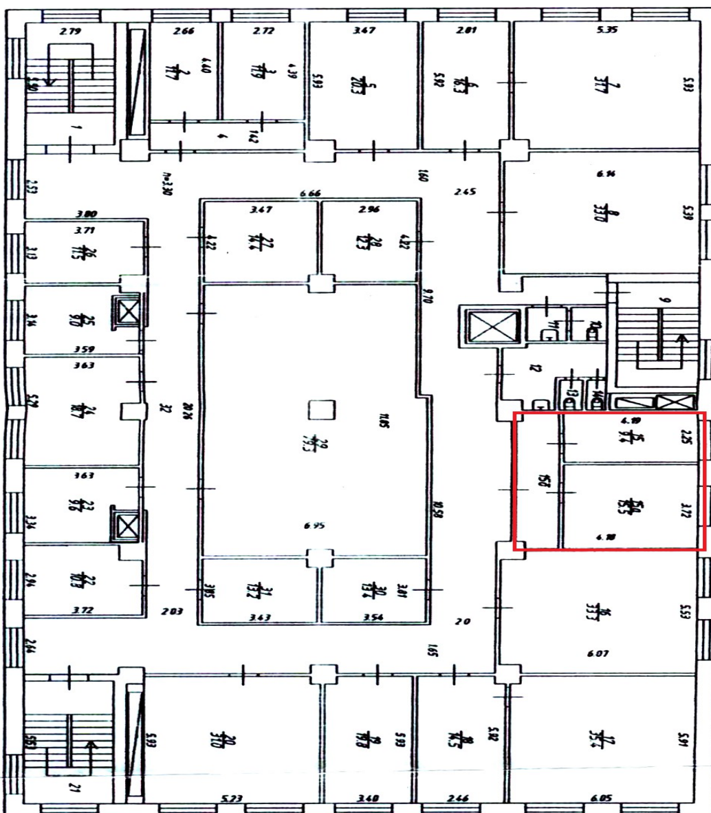
План 3 этажа
